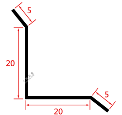
L型内角 ● 244 cm
